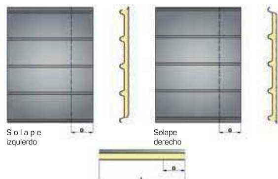
Detalle sistema de solape
