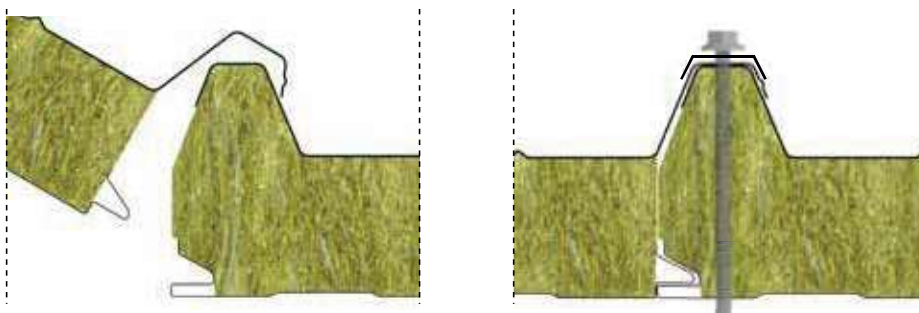
Modalidad de fijación del Panel
